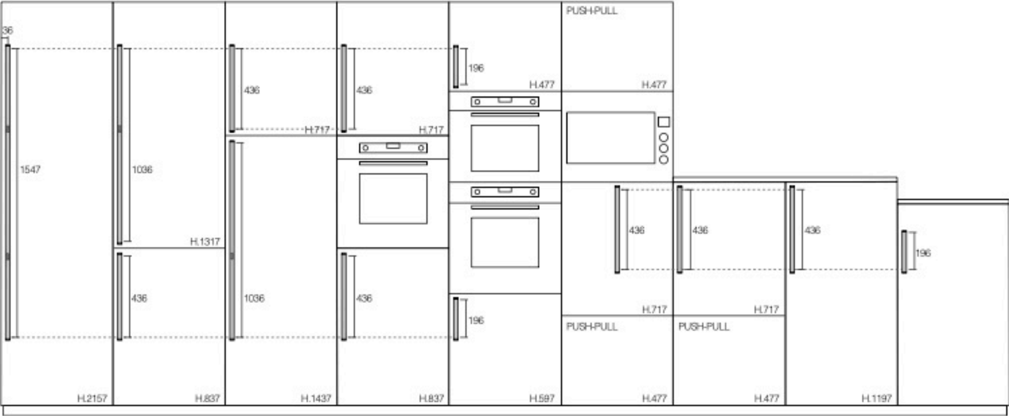
COLONNE ZOCCOLO H.6 H.6 PLINTH COLUMNS
