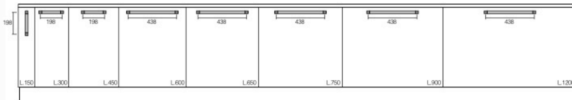
BASI ZOCCOLO H.6 e H.13
